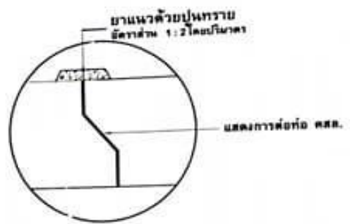
รูปตัดแสดงการยานแนวรอยต่อท่อ
