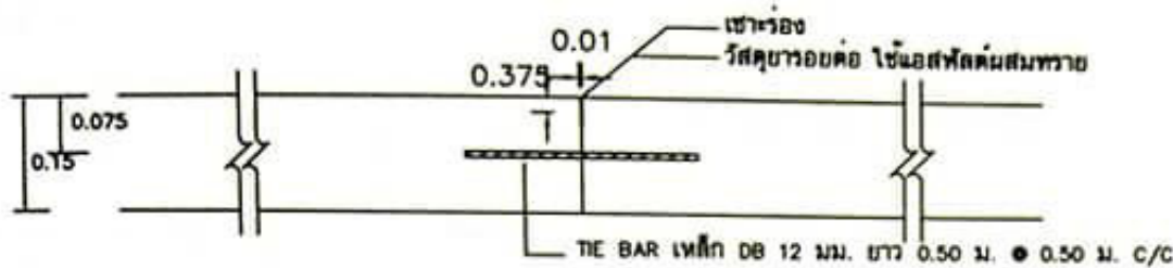
ขยายรอยต่อ LONGITUDINAL JOINT
