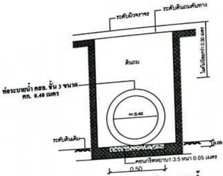
รูปตัดแสดงการวางท่อระบายน้ำ
